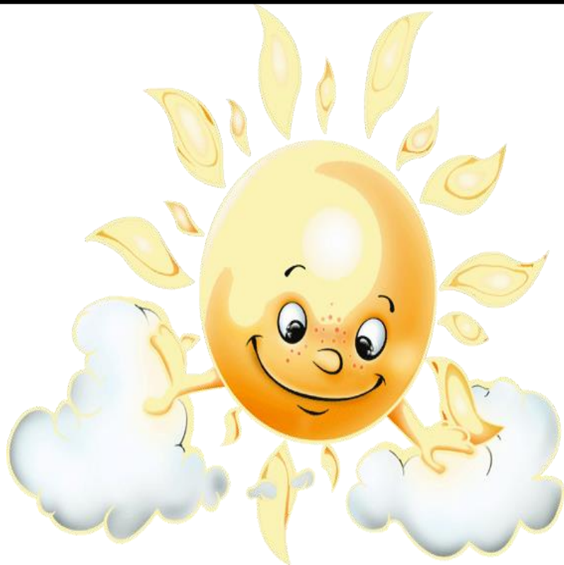
Солнце – тепло .
